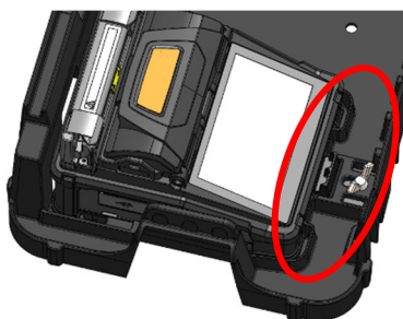
2: 拉开固定部件，将熔接机正确地放在 WT-18 上。
