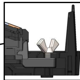
3: 推动固定部件，并完全拧紧拇指螺丝。
