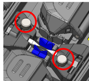
电极棒的固定板螺丝
